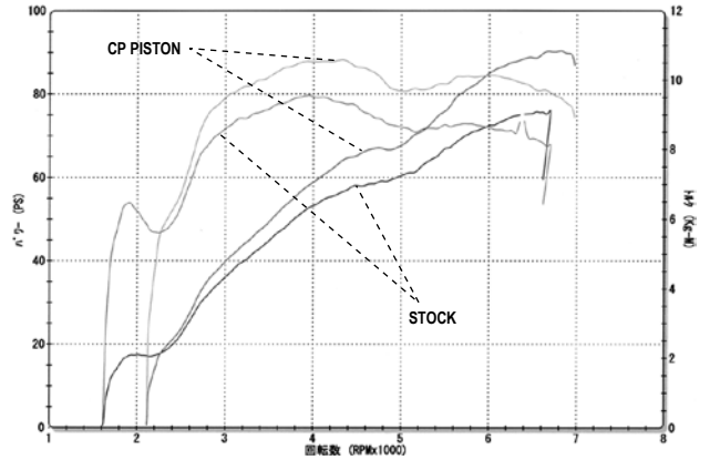
純正ピストンとCP PISTON(Evolution用)の比較
