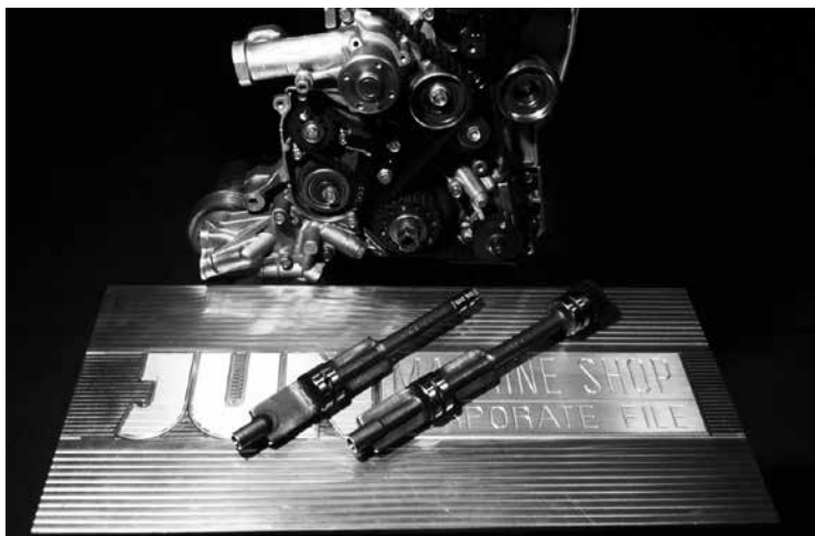
4G63ブロックバルンサーシャフトカット加工
